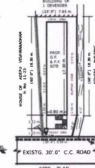
SITE - PLAN SCALE: 1:200 cm.
