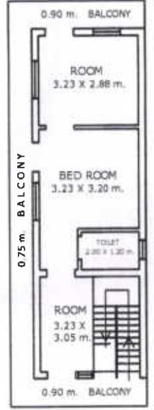
PROP. F. F. PLAN
