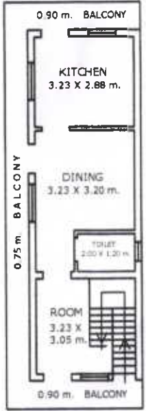
PROP. G. F. PLAN
