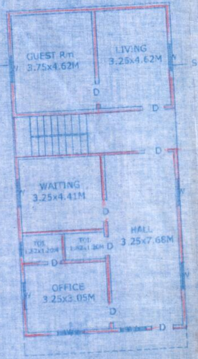
PROP. F.F. PLAN
