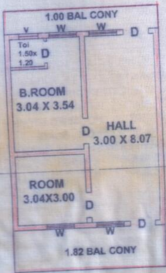
F.F. PLAN
