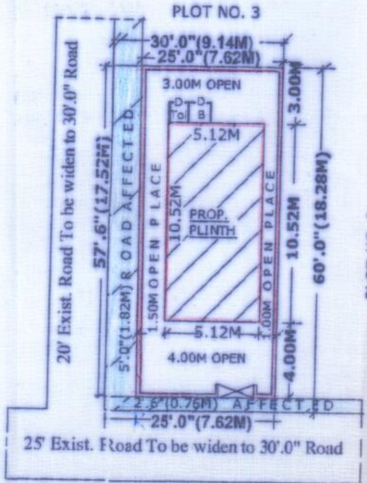
SITE PLAN SCALE: 1:200 CM
