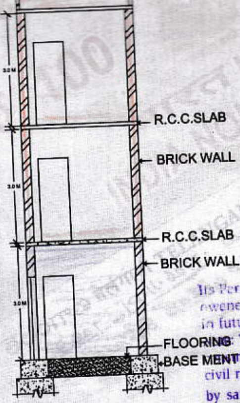
SECTION A-B
