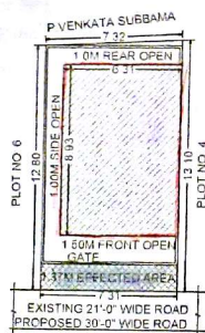
SITE PLAN SCALE: 1:200
